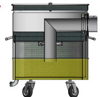
Integrierter und fahrbarer INERT-Nassabscheider in Edelstahl
