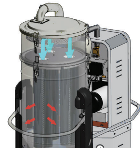
Vollautomatische Patronenfilteranlage mit Wechselreinigung
